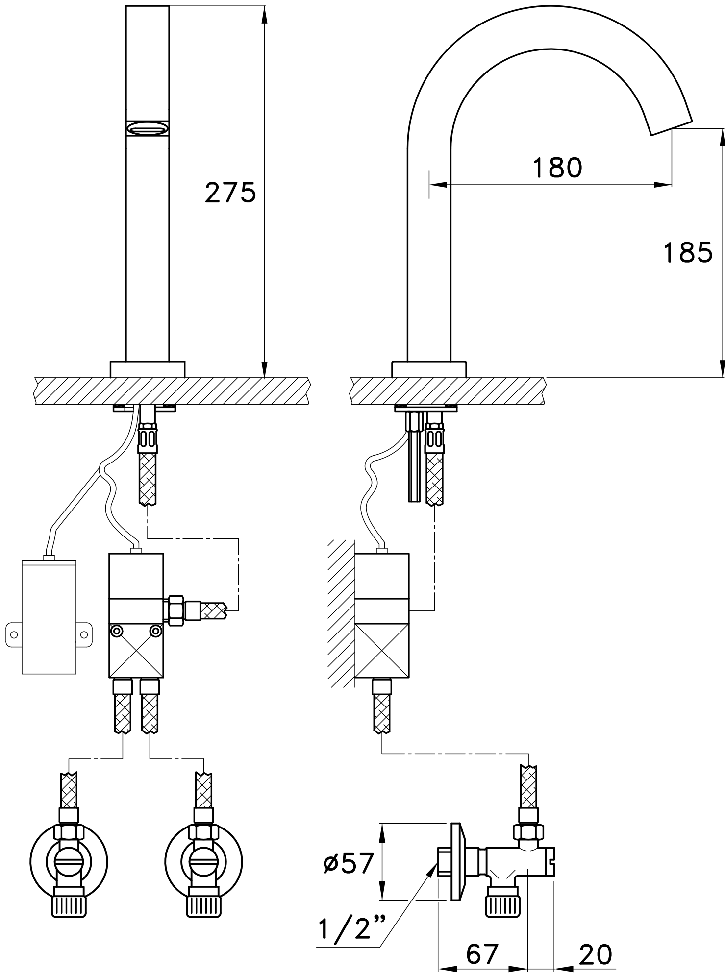
TELETRON QUADRO (2-acque)
